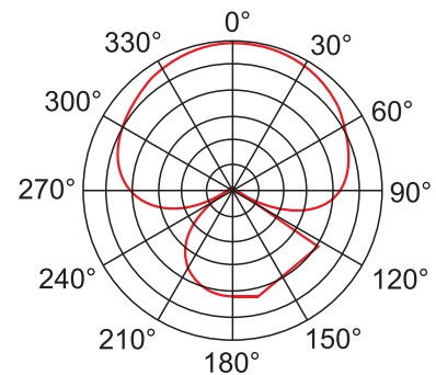
Cardiíde (em 1KHz)
