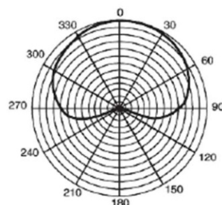
Direcionalidade Cardioide (a 1 kHz)
